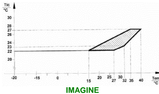
Figura nr. 4*) - Curba de reglaj pentru temperatura interioară prescrisă
